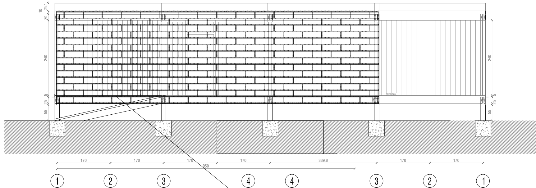
CORTE 11 ESC 1/25
