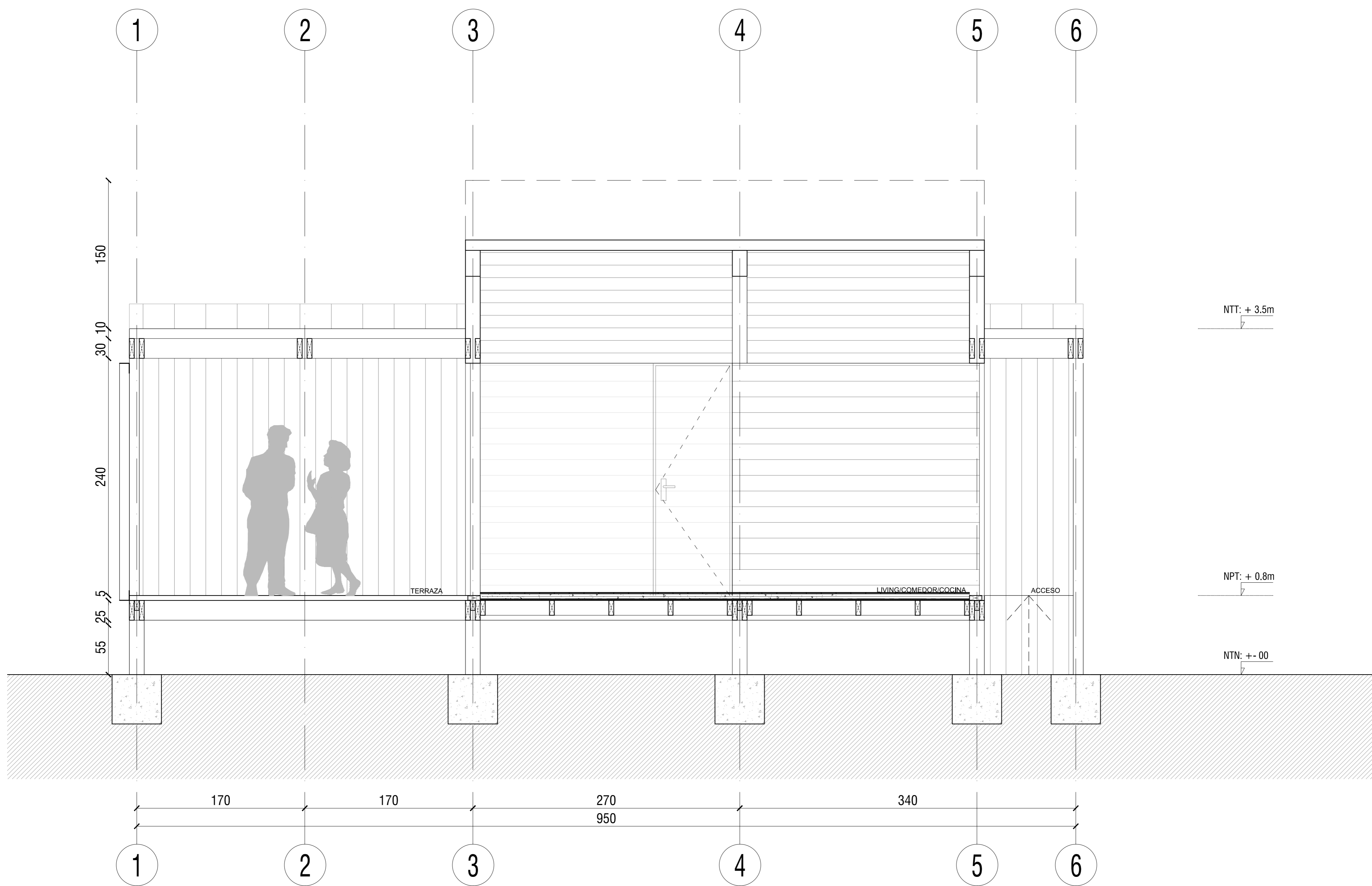
CORTE 11 ESC 1/25
