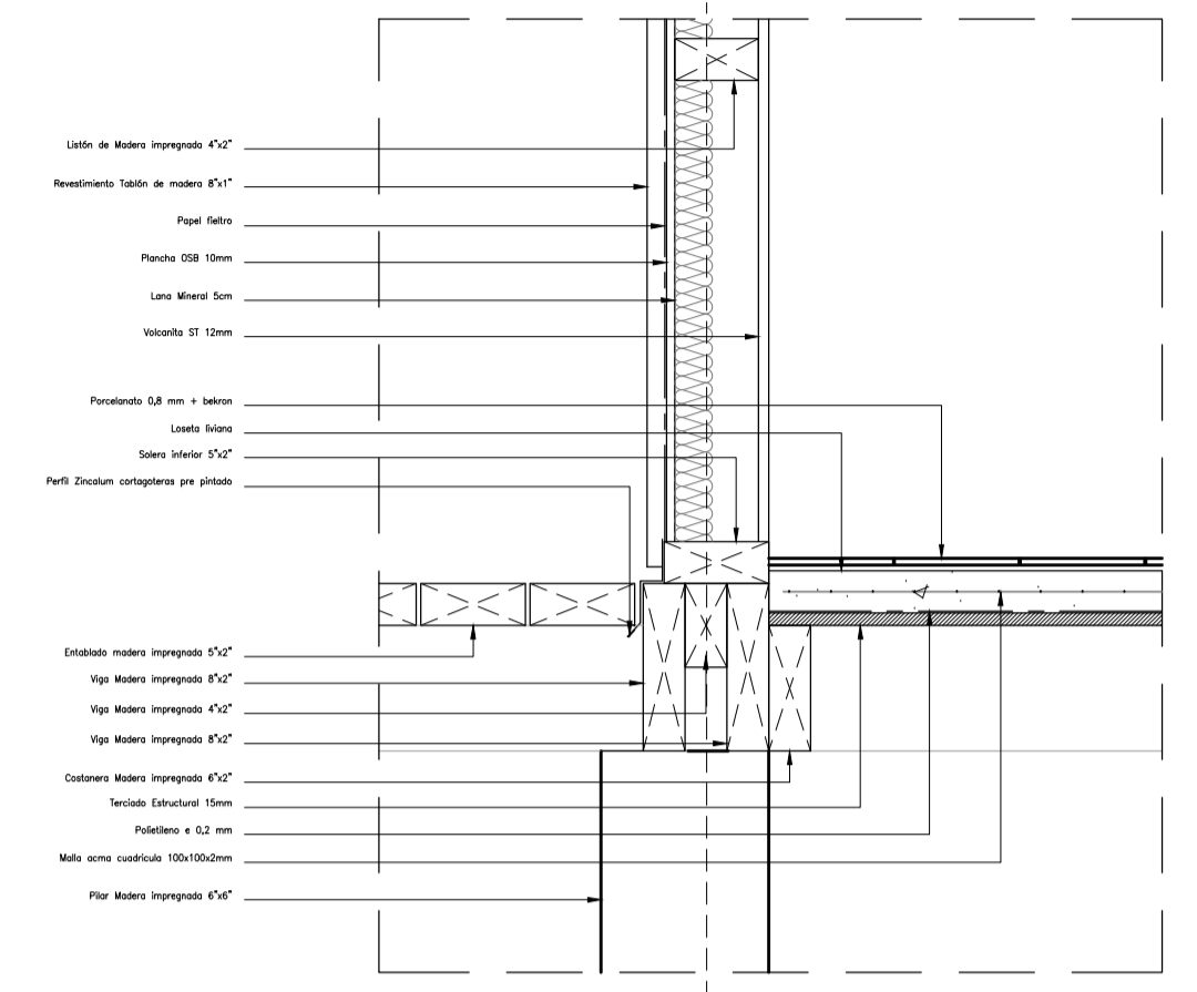
DETALLE MURO TIPO ESC 1/5
